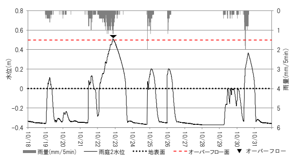
図6 雨量と水位変化(雨庭2)
