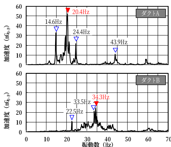
図1 空調ダクト振動の周波数分析結果例
