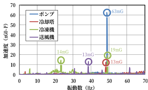
図12 設備機器の振動測定例
