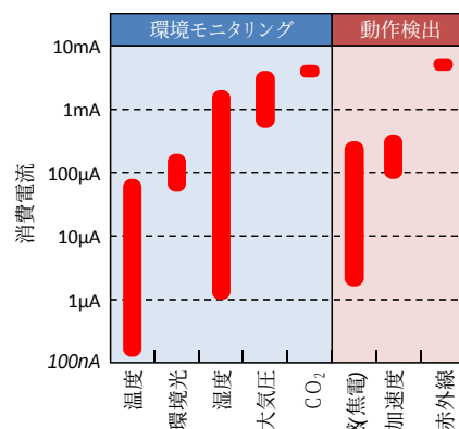
図10 各種センサの消費電流
