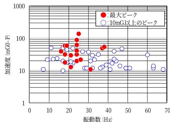
図2 空調ダクトの振動分布
