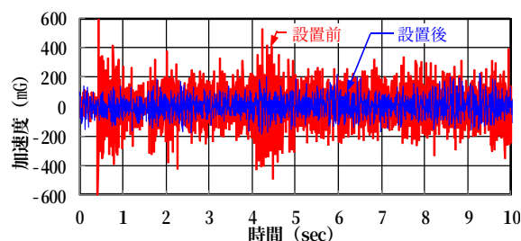
図8 発電デバイス設置前後のダクト振動の波形
