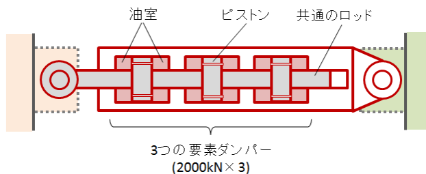
図4 高減衰オイルダンパーの基本構成
