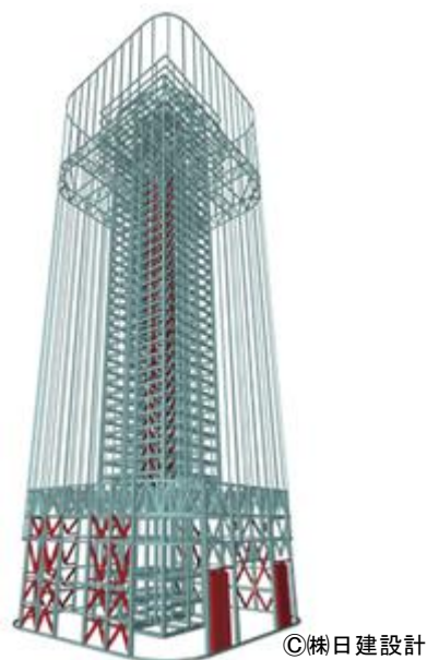
図 9 中之島フェスティバルタワー・ウエスト 構造システム概念図
