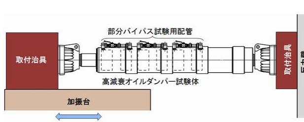
図 6 加力概念図
