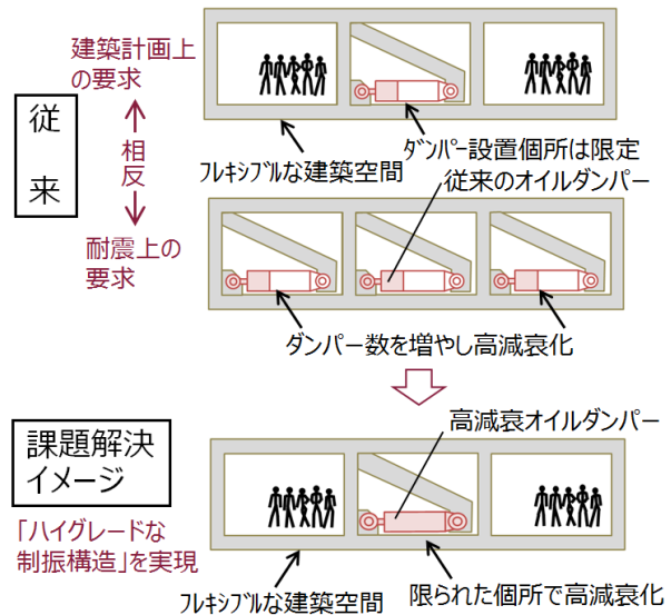
図1 高減衰オイルダンパーによる課題解決のイメージ
